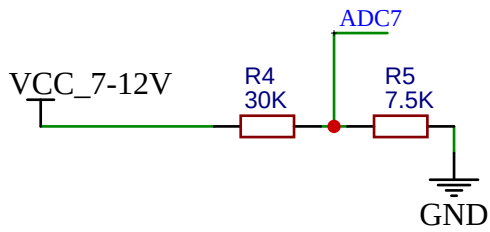
电池电压检测 (0-5V)
