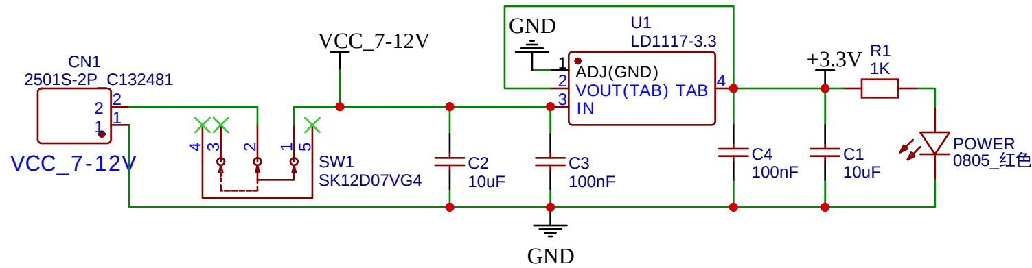
3.3V电源
