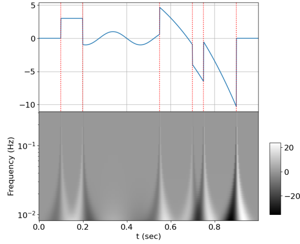
FIGURE 48 – En haut: signal régulier par morceaux. En bas: carte avec en abscisse le paramètre de de translation et en ordonnée la fréquence (grande fréquence = petite échelle). Ici on a utilisé l'ondelette réelle en forme de chapeau mexicain ("mexh" pour la librairie PyWavelets.)
