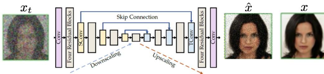
FIGURE 33 – Réseau U-Net utilisé comme débruiteur.
