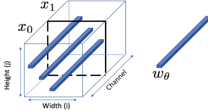
FIGURE 24 – Schématisation de l’opération de convolution 1 \times 1 (vecteur w_\theta de dimension C ) qui agit sur les canaux identiquement sur les pixels H \times W .
