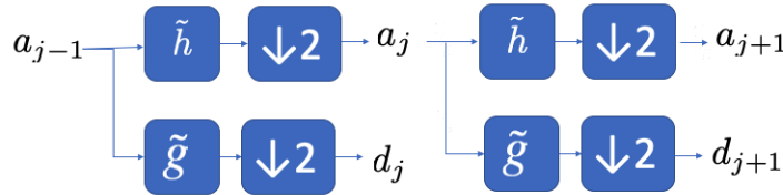
FIGURE 59 – À partir des coefficients d'approximation a_{j-1} , on obtient les coefficients d'approximation a_j et de détails d_j , par filtrage et sous-échantillonnage.
