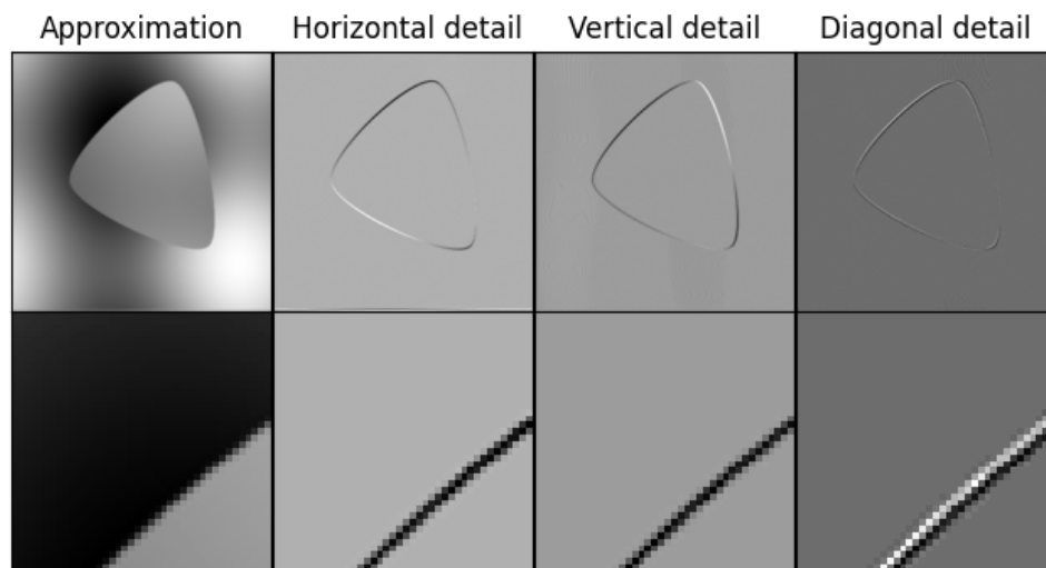
FIGURE 66 – Décomposition en ondelettes ("db1", 1 seul niveau) d'une image constituée d'un fond régulier et d'une forme elle-même régulière enfermant un fond tout aussi régulier. En bas: un simple zoom sur le bord de la forme dans la partie supérieure gauche.
