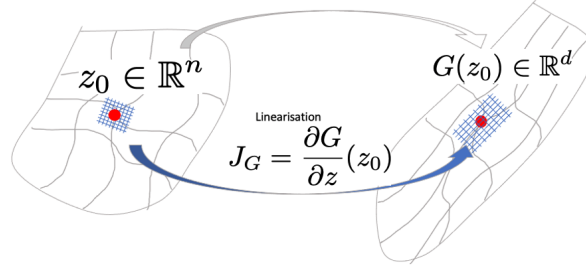
FIGURE 17 – Illustration de la fonction du Jacobien du générateur G entre l'espace des variables latentes ( z ) et l'espace des données ( x ).
