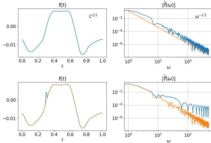
FIGURE 45 – Exemple de traitement par Fourier d'une fonction de régularité C^{2.5} (en haut) à laquelle on ajoute un petit pic localisé en temps (en bas). On remarque que dans le premier cas la décroissance des coefficients de Fourier renseigne bien de la régularité de la fonction (voir la courbe orange \propto \omega^{-2.5} sur le spectre), et dans le second cas le spectre à haute fréquence est dominé par celui de la perturbation (en orange le spectre initial).
