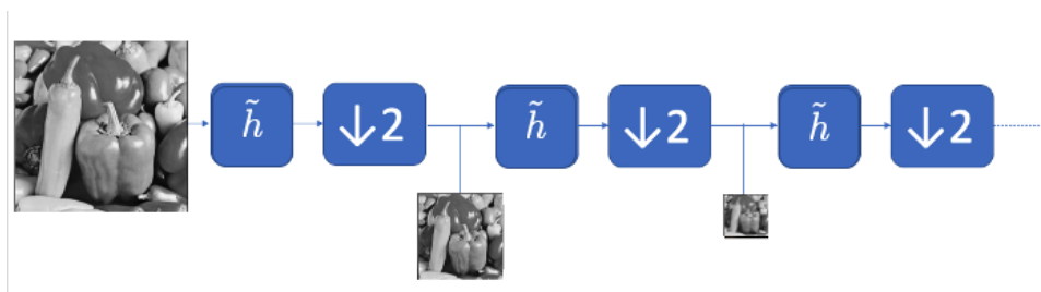
FIGURE 58 – Illustration de l'obtention d'approximations de plus en plus à grande échelle par une cascade de convolutions et sous-échantillonnages d'un facteur 2.
