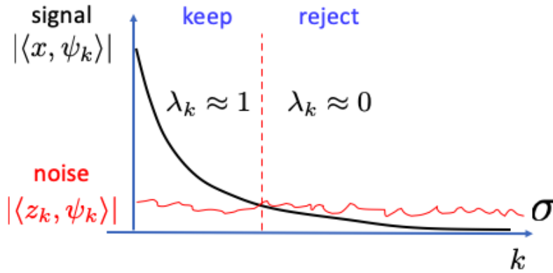
FIGURE 69 – Sélection des coefficients dans la base obtenue par le réseau selon les valeurs propres de l'opérateur.
