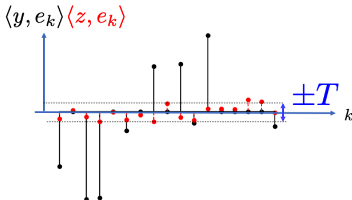
FIGURE 43 – Distribution des produits scalaires du signal bruité y et du bruit z . Un seuillage en \pm T peut enlever le bruit sans trop dénaturer les caractéristiques du signal x .
