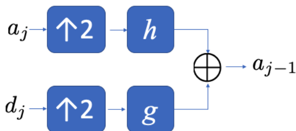
FIGURE 61 – À partir des coefficients a_j et d_j , on peut reconstruire les coefficients a_{j-1} la dernière faisant apparaître le grossissement d'un facteur 2 des tailles des coefficients a_j et d_j par insertion de 0 avant le filtrage.
