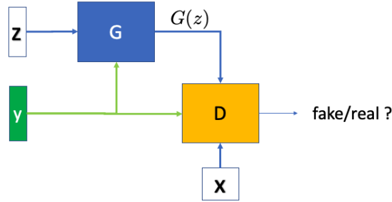
FIGURE 20 – Schématisation d'un GAN conditionnel: par rapport au schéma de la figure 6, on ajoute l'information y à l'entrée du générateur et du discriminateur.
