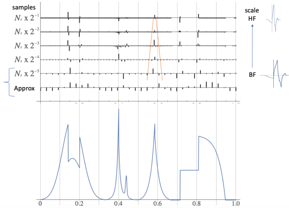
FIGURE 54 – De bas en haut: la fonction échantillonnée pour donner 2^S = 1024 échantillons ( S = 10 ), puis par décomposition successive avec l'ondelette de "Db2" on aboutit aux coefficients d'approximation basse fréquence au nombre de 2^{S-5} = 32 et aux coefficients de détails à la même échelle, puis on dispose des coefficients de détails de plus en plus de hautes fréquences jusqu'à aboutir à ceux au nombre de 2^{S-1} = 512 . Notons que la plupart des coefficients de détails sont quasiment nuls, et que les coefficients de détails les plus importants se concentrent aux discontinuités de la fonction d'origine dans le cône du théorème 14 (en orange; voir Th. 12 Cours 2021). Les échelles verticales ne sont pas les mêmes pour chaque lots de coefficients. Nb. la présentation au vidéoprojecteur de S. Mallat est dans l'ordre inverse pour l'agencement des coefficients de détails allant de haut en bas, des basses fréquences aux hautes fréquences. De plus, l'approximation de basse résolution n'est pas représentée..
