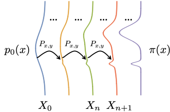
FIGURE 15 – Évolution de la distribution initiale p_0(x) vers la distribution cible (ici notée \pi(x) ) par application de la matrice de transition P_{x,y} de la chaîne de Markov.
