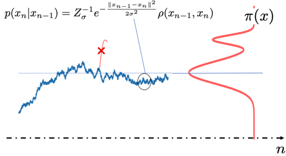
FIGURE 16 – Cas problématique d’une distribution cible \pi = p_\theta multi-modale ( U_\theta(x) non convexe et un noyau Q(x, y) gaussien avec un \sigma trop petit.
