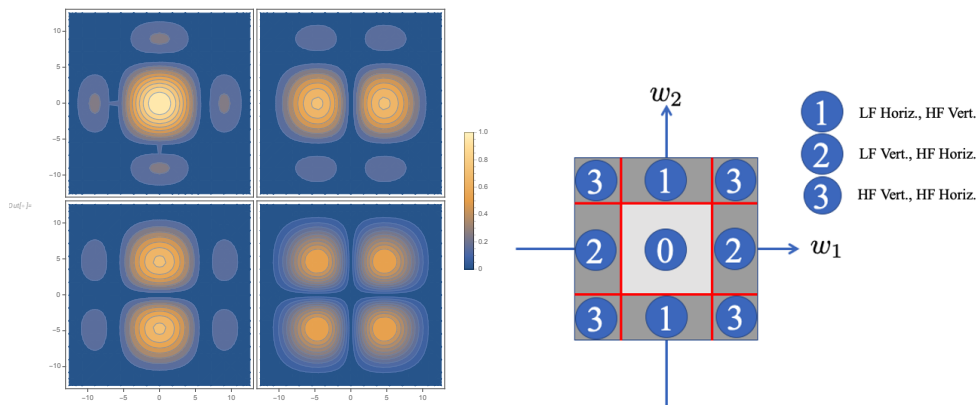
FIGURE 57 – À gauche: Couverture du plan de Fourier par les différents types d'ondelettes 2D construites à partir des ondelettes 1D (filtre passe bas en haut à gauche, les autres panels correspondant aux filtres directionnels passe bandes; "LF": low frequency, "HF": high frequency). À droite: schéma correspondant avec le filtre passe-bas ("0") et les différents filtres passe-bandes détectant des détails sur les variations rapides (transitoires) dans 3 directions différentes. L'ondelette de base est celle de Haar ("db1").
