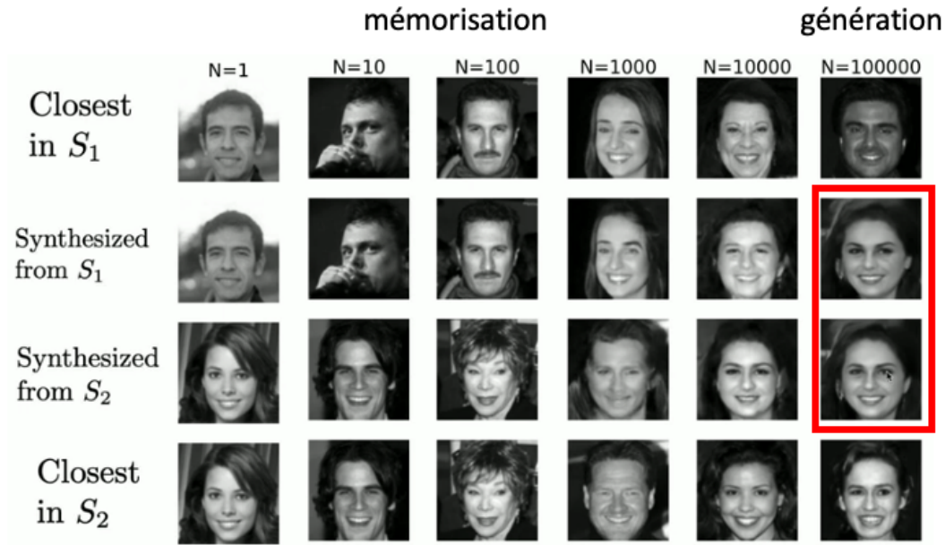
FIGURE 13 – Deux modèles génératifs S_1 et S_2 sont entraînés avec deux sous-lots issus de la même base de données d’images de visages ( 80 \times 80 pixels) sans recouvrement et chacune de taille N . On donne ensuite la même image de bruit aux deux modèles afin de synthétiser une nouvelle image. On peut trouver l’image de la base de donnée qui approcherait au mieux cette image synthétisée. Tant que N < O(10,000) , S_1 et S_2 produisent des images différentes, et ressemblant d’autant plus à une image de la base de données que N est petit. Dès que N = 100,000 , les images synthétisées par S_1 et S_2 sont d’une part (quasi-)identiques et d’autre par différentes des images les plus proches des deux bases de données. On assiste bien à une transition vers un modèle qui généralise bien: il a appris la distribution de probabilité p(x) .
