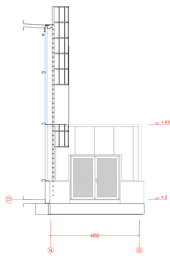
AANZICHT as-13
