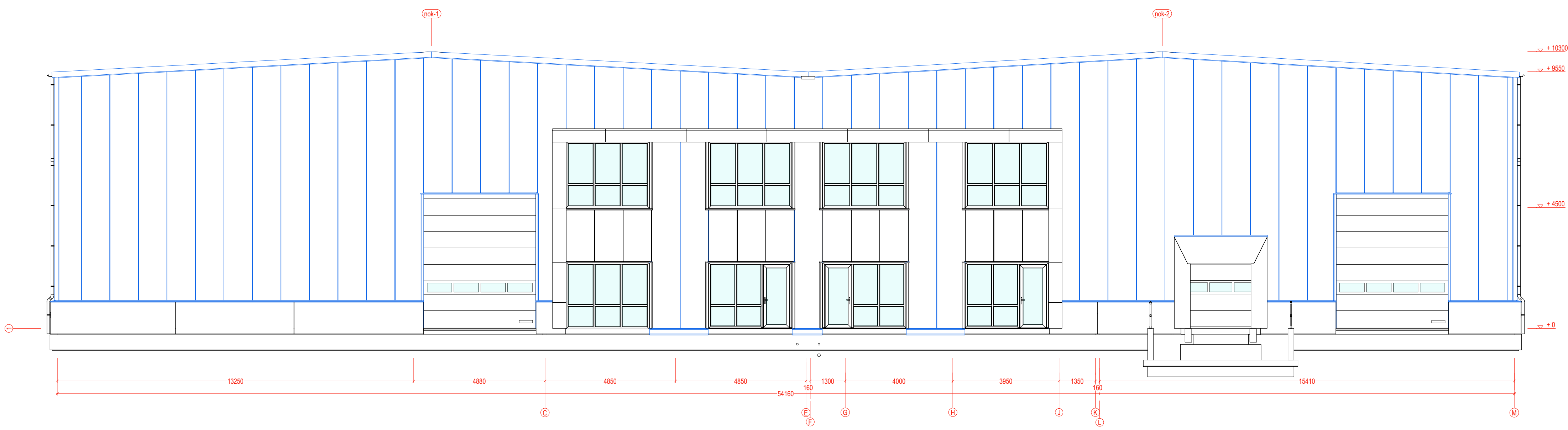
AANZICHT as-1
