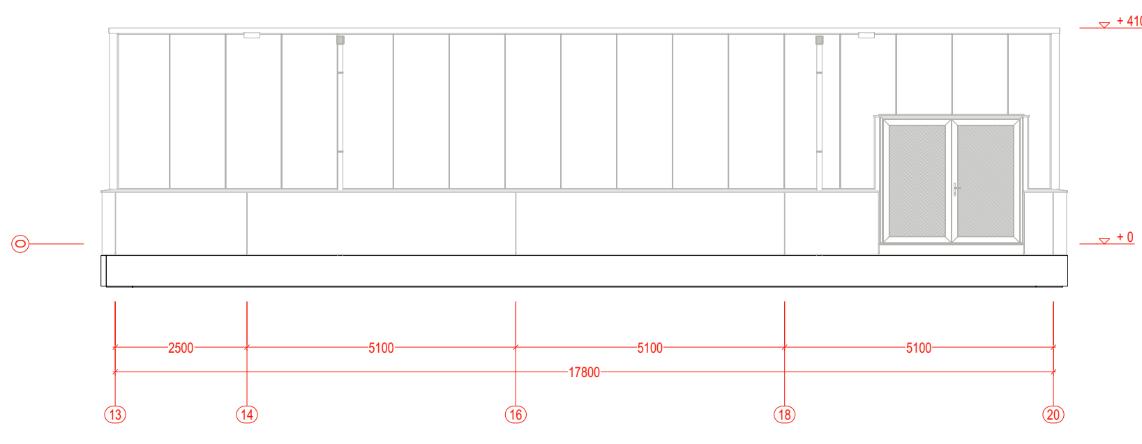
AANZICHT as-O
