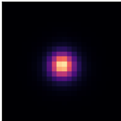
ImplicitPSF (ours)
