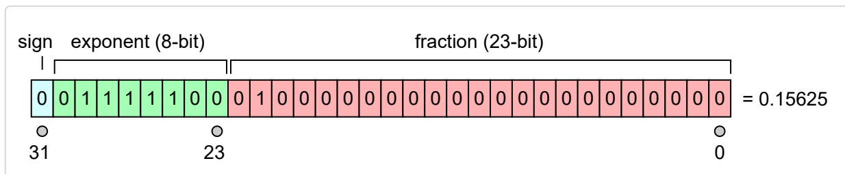
图源: IEEE 754 Single Floating Point Format, Wikimedia Commons, CC BY 3.0。
