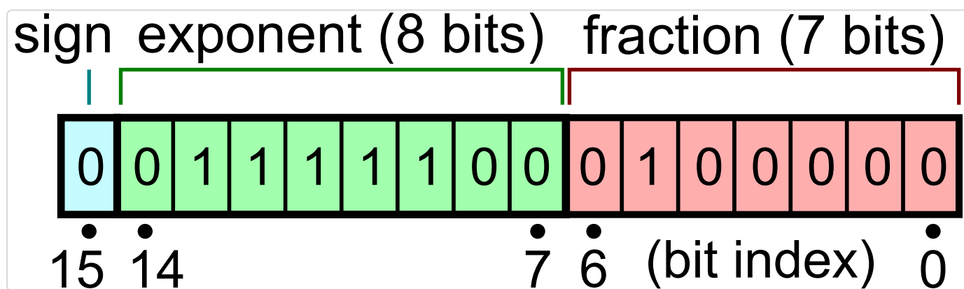
图源: Bfloat16 format, Wikimedia Commons, CC BY-SA 4.0。三张图对照看 s / e / m 的位数分配——这就是 Q7 那道「fp16 与 bf16 差在哪」的全部答案: bf16 用尾数换 range (8 位指数 = fp32), fp16 用 range 换精度 (10 位尾数)。
