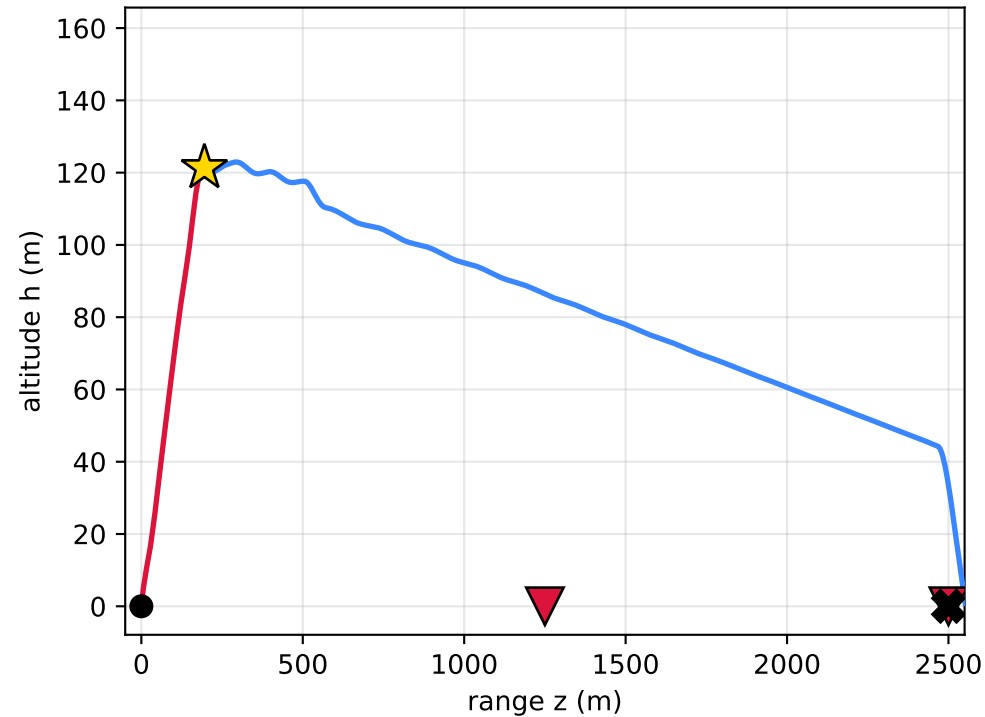
SSE
