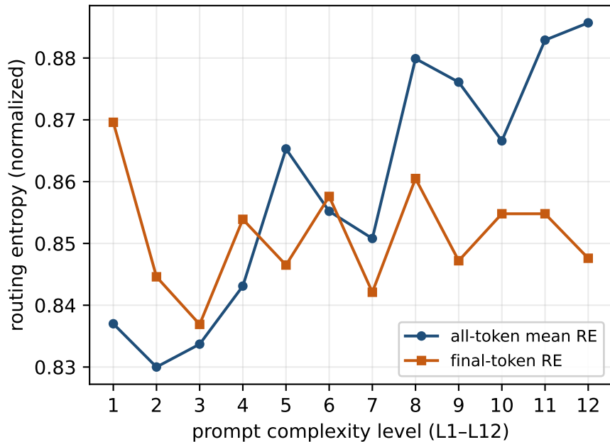
DeepSeek V3.1
