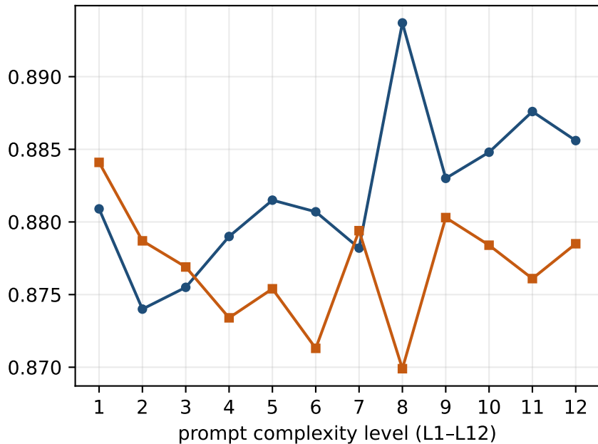
Qwen 397B
