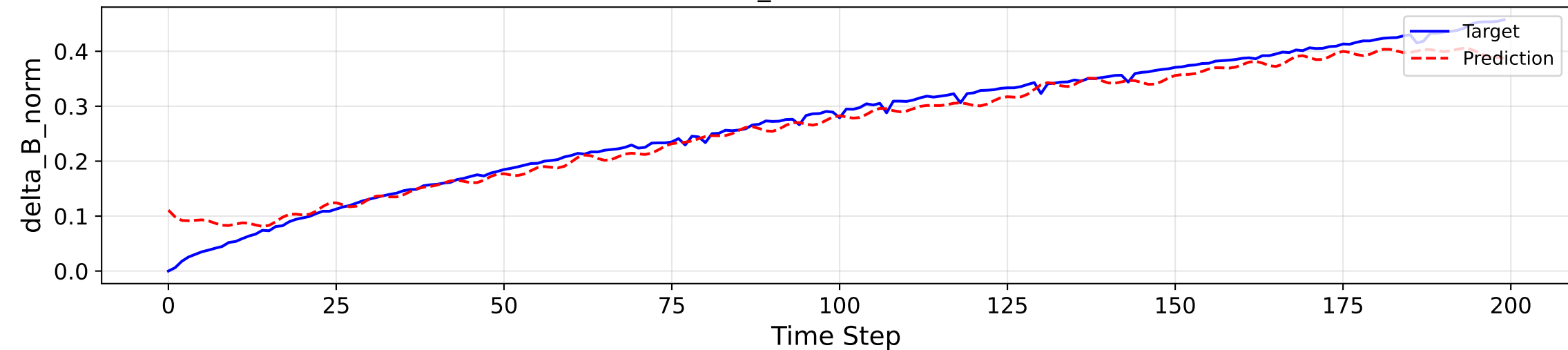
delta_B (MAE: 0.0169)
