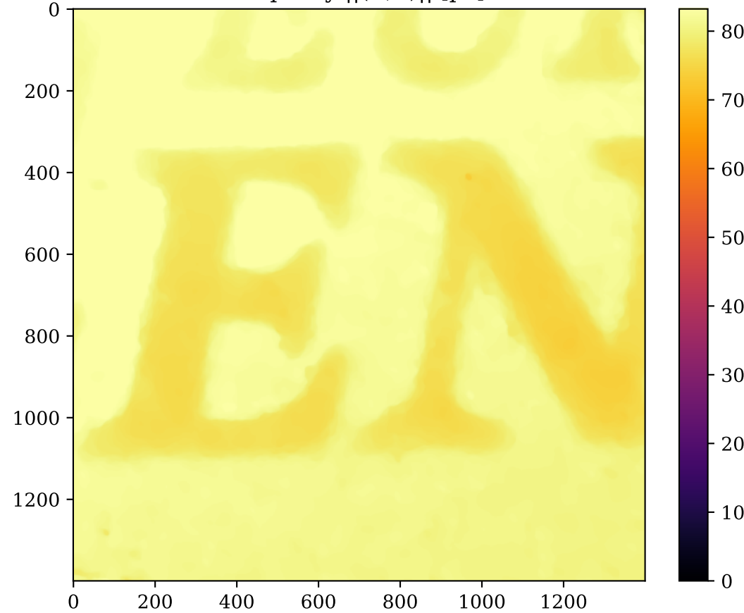
Zernike O(2)+d(2) Z [mm]
