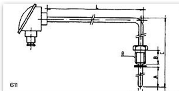
Caña pirométrica acodada. Fijación por raccord libre y arandela de tope.
