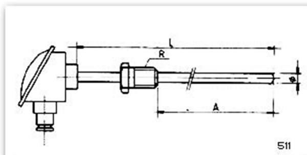
Caña pirométrica recta. Fijación por raccord soldado.
