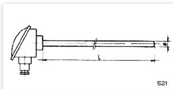
Caña pirométrica recta sin fijación.
