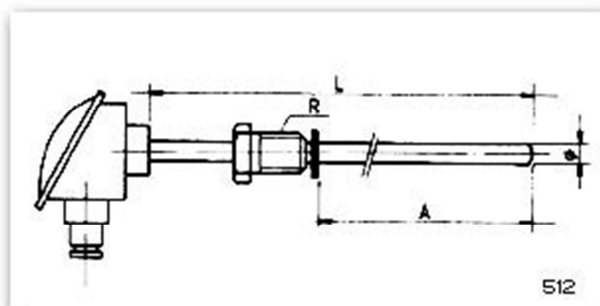
Caña pirométrica recta. Fijación por raccord libre con arandela tope soldada.
