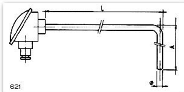
Caña pirométrica acodada sin fijación.
