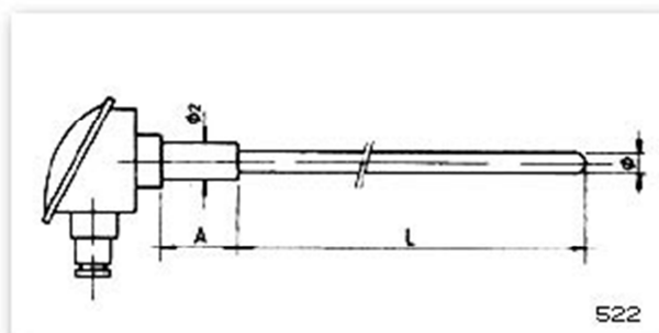
Caña pirométrica recta sin fijación. Protección simple material cerámico compacto.
