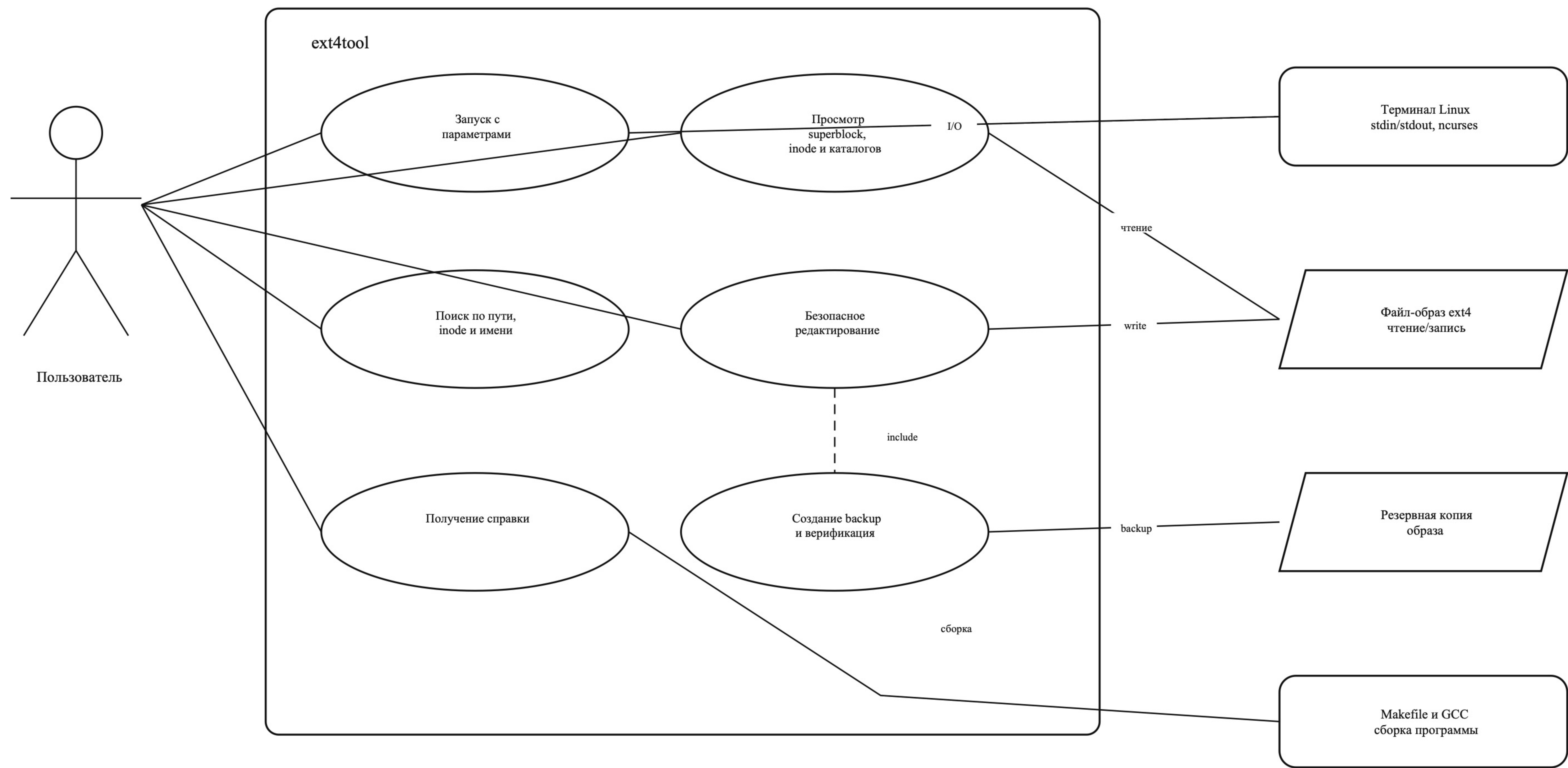
Схема показывает пользовательские сценарии и внешние объекты, с которыми взаимодействует программа.
