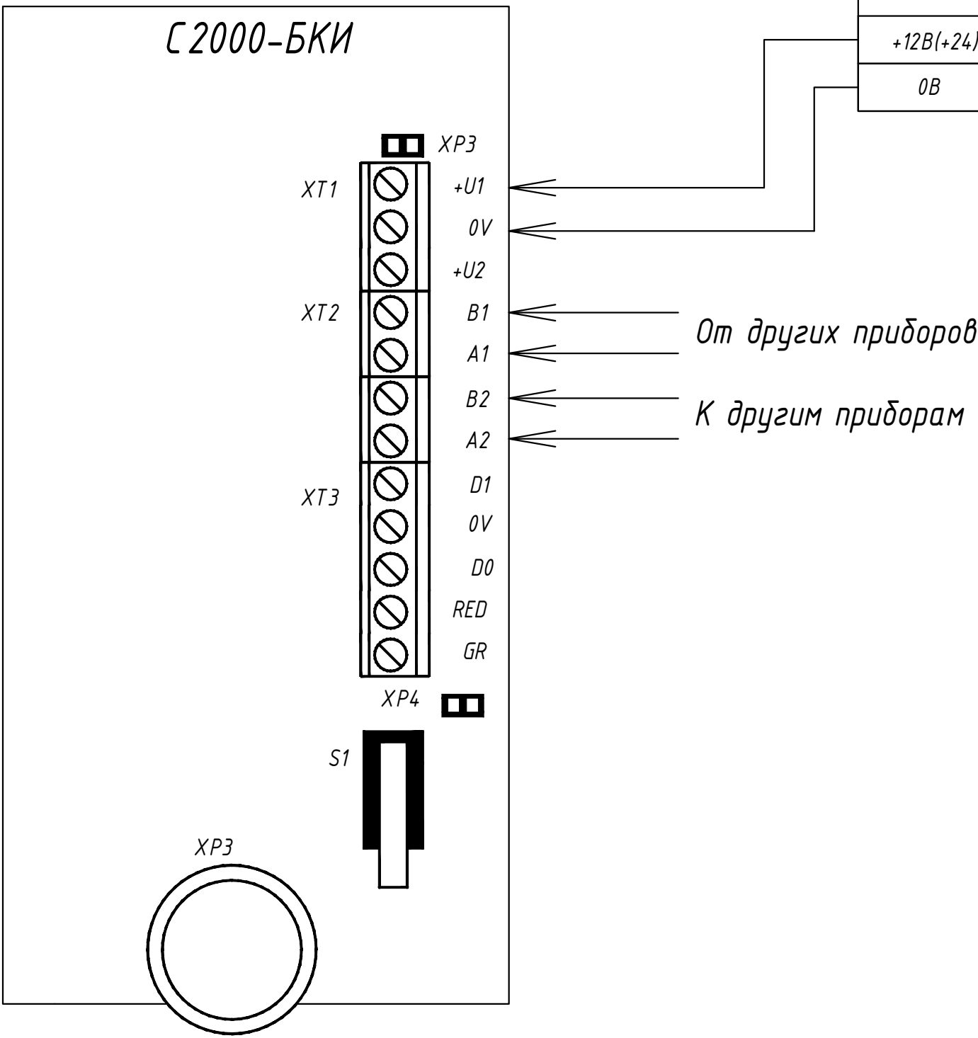
Источник питания Схема подключения "С2000-БКИ"
