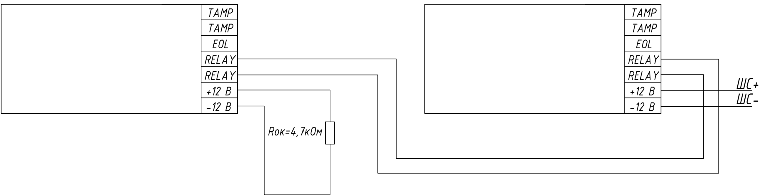
Схема подключения извещателя инфракрасного объёмного ИНС-105
