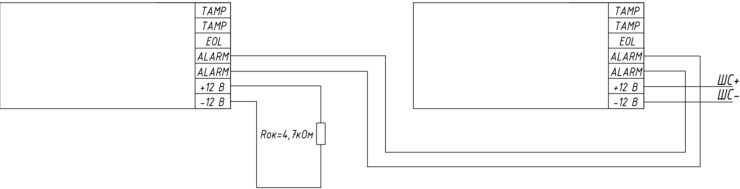
Схема подключения извещателя инфракрасного поверхностного ИНС-106
