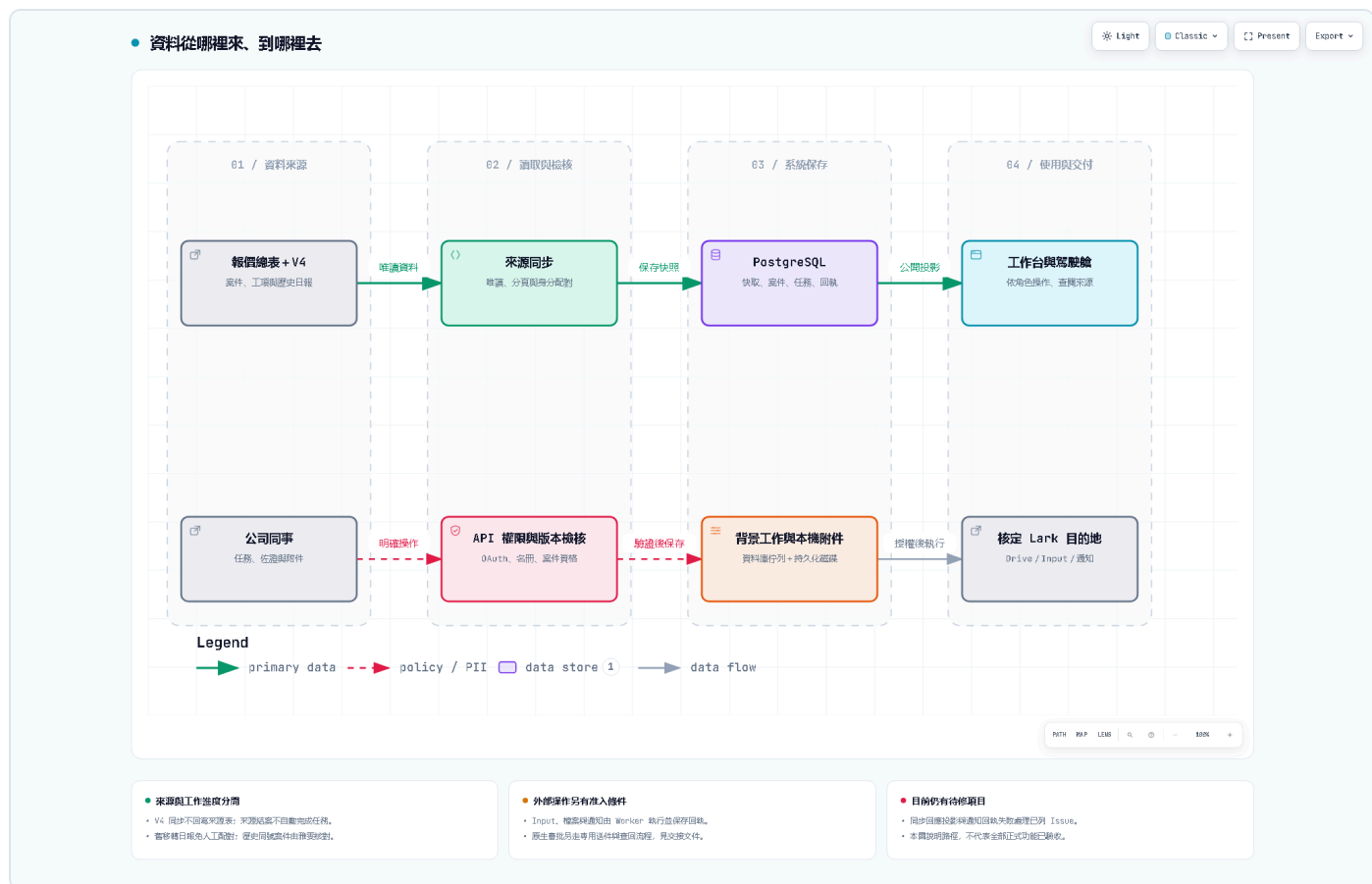
資料流與風險所在路徑
