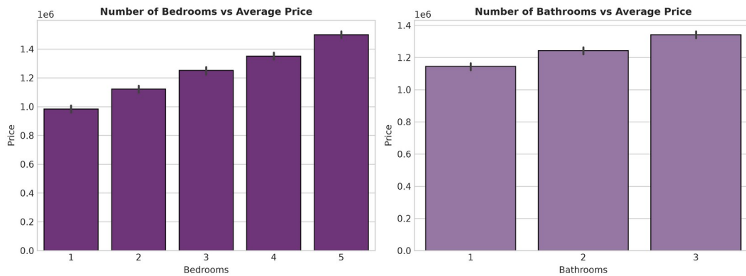
Hình 8.3. Mối quan hệ giữa Số phòng ngủ, Số phòng tắm và Giá nhà.
