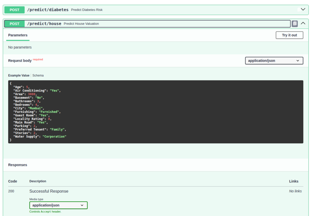
Hình 8.7. Kết quả gọi API định giá bất động sản ( /predict/house ) trên Swagger UI.
