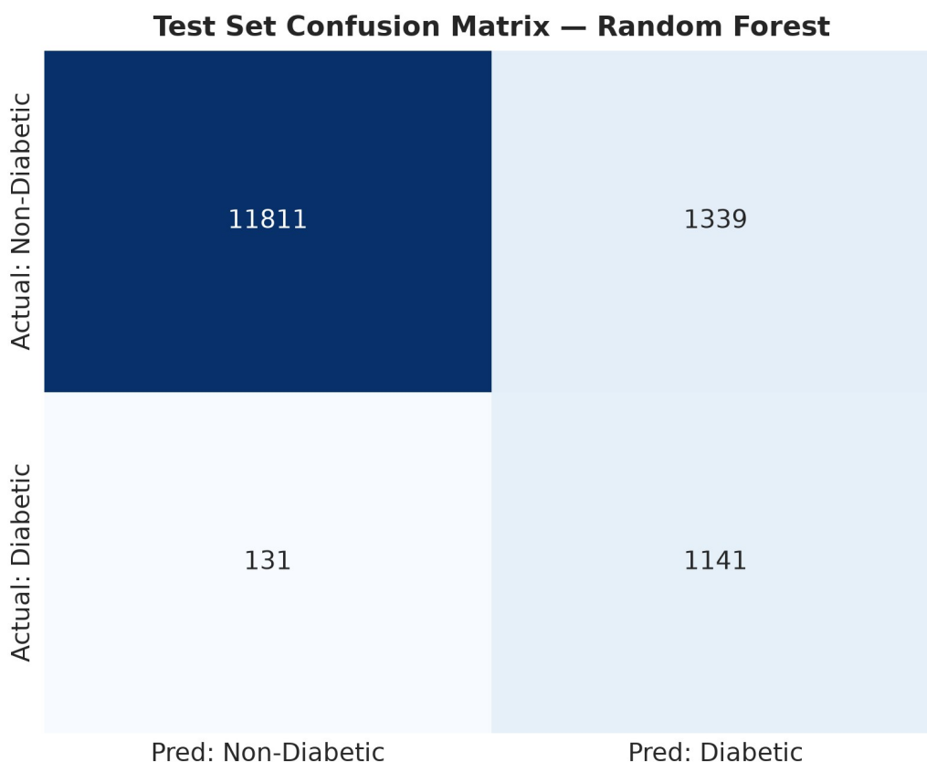
Hình 7.7. Ma trận nhầm lẫn ( Confusion Matrix ) của mô hình Random Forest trên tập Test độc lập.
