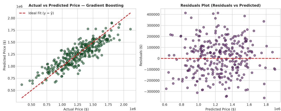
Hình 8.6. Đồ thị Giá thực tế so với Giá dự đoán và Phân bố phần dư (Residuals) trên tập Test.
