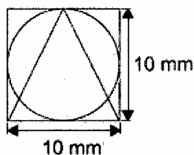
Figure 2 : Dimensions des symboles pour l'étiquetage de sécurité
