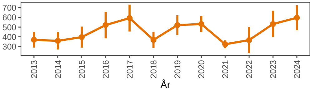
Nedbørsum
