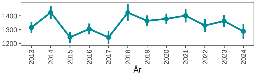
Temperatursum
