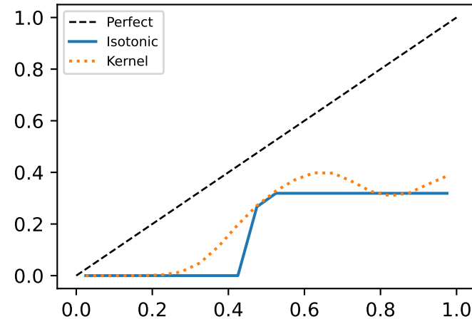
moral_scenarios ECE=0.483
