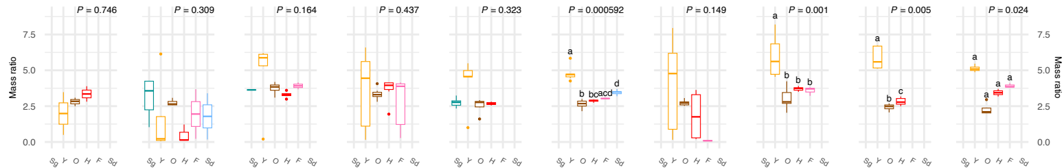
Chlorophyll a:b
