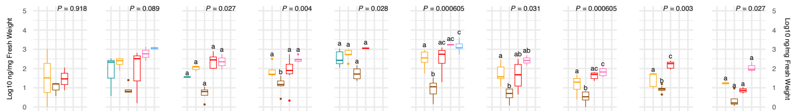
Chlorophyll b
