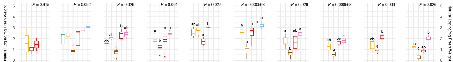
Chlorophyll b
