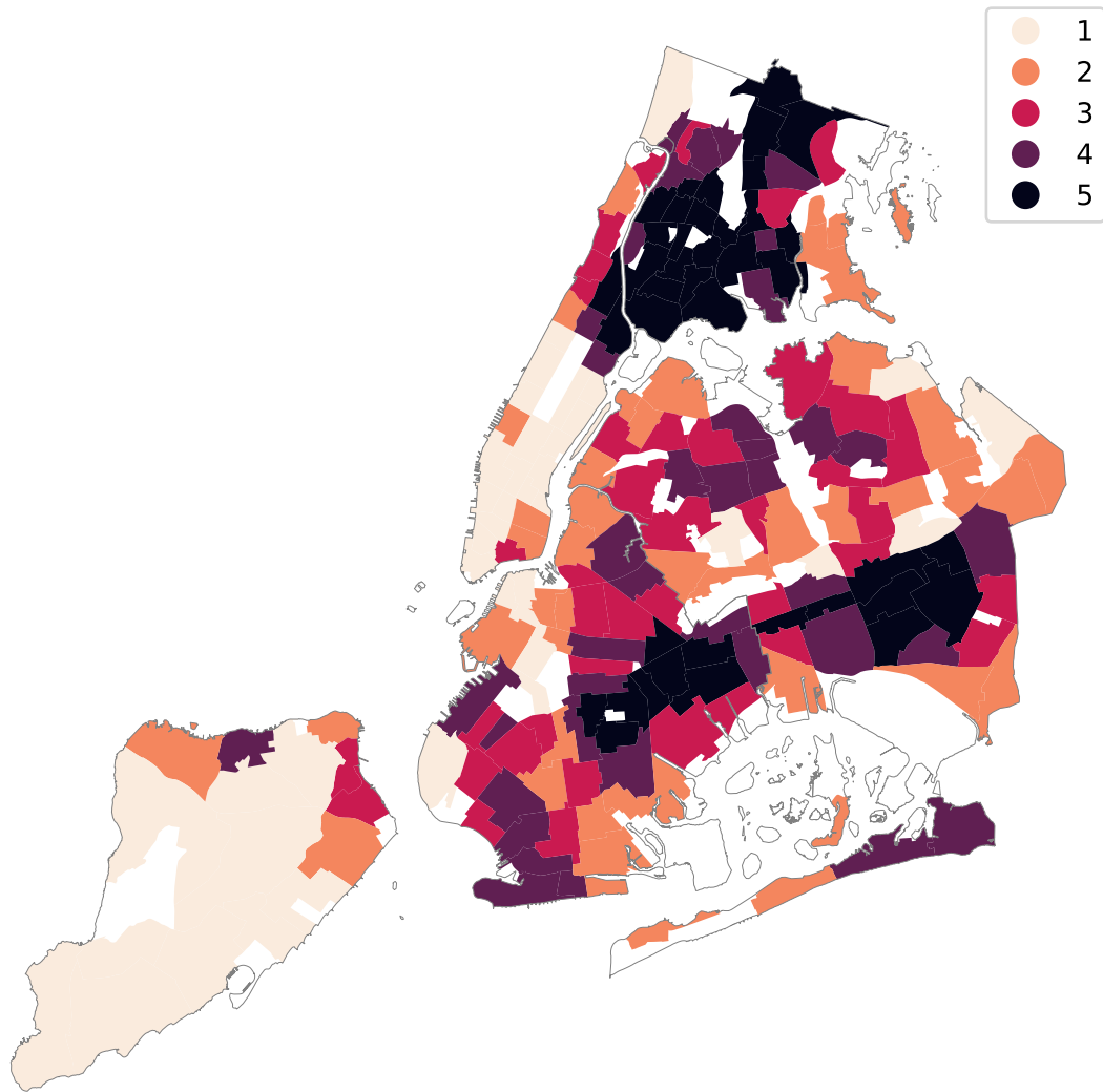
HVI: minority
