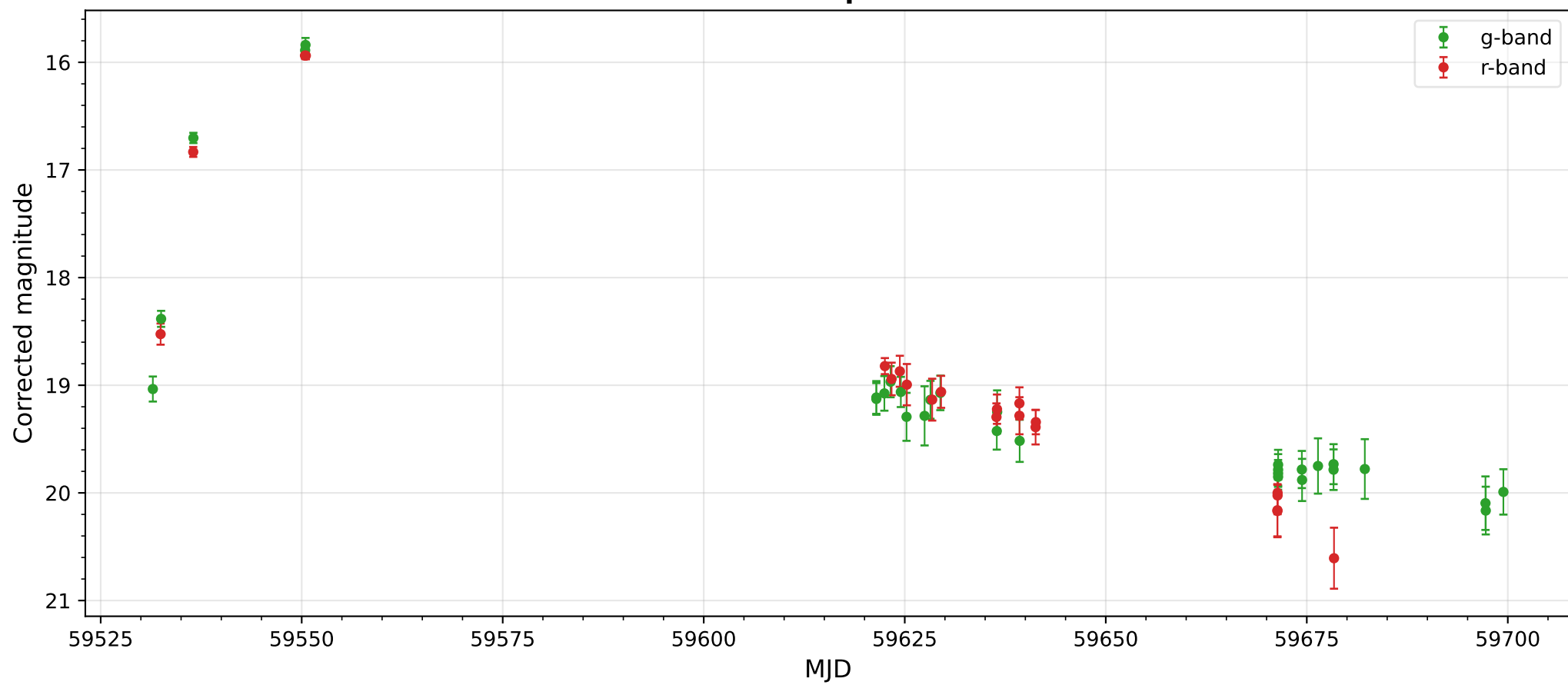
ZTF20aapchqy
