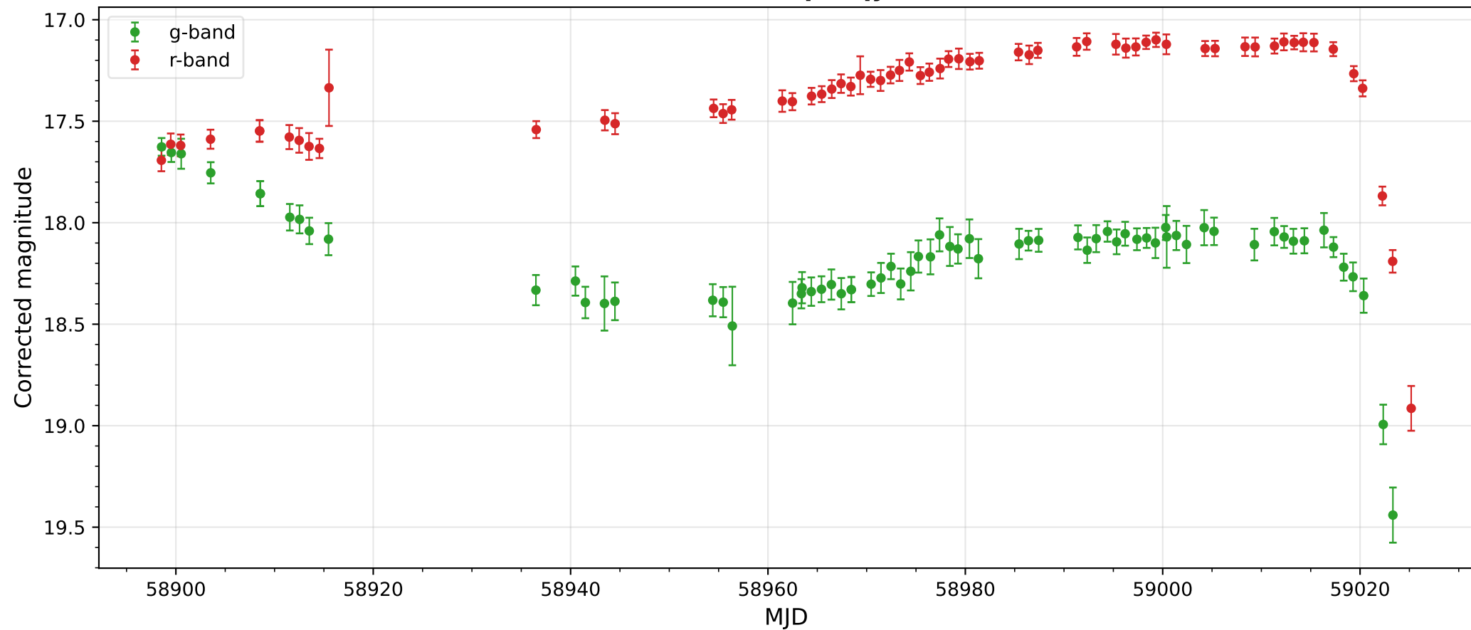
ZTF24aahkzvn
