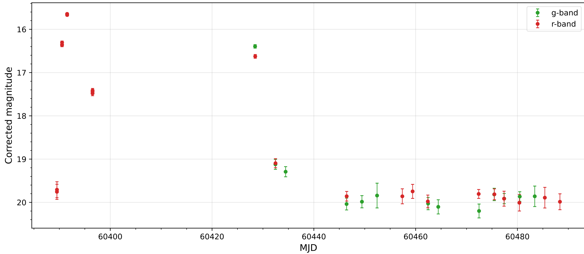
ZTF24aahkzvn
