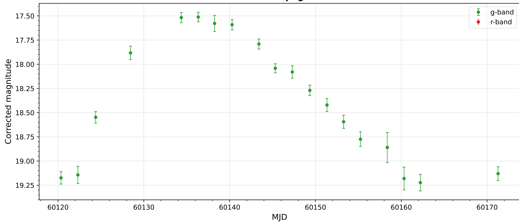
ZTF23aapogvn
