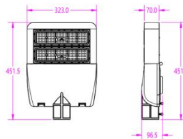
Dimensions
