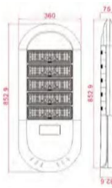
Dimensions
