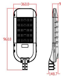
Dimensions
