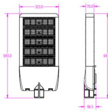
Dimensions
