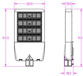
Dimensions
