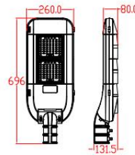
Dimensions
