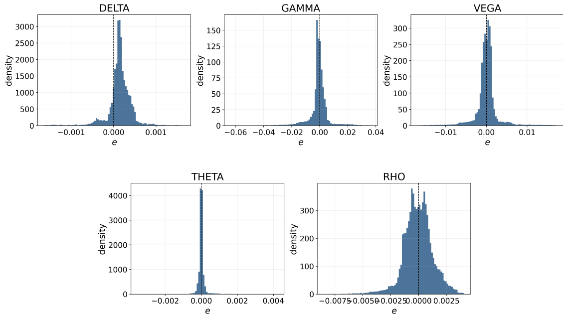
Fig. 5.10. Sobolev PINN Greek error histograms.
