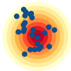
unverzerrt, hohe Varianz
