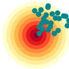
verzerrt, hohe Varianz
