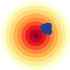
verzerrt, niedrige Varianz
