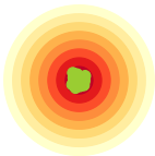
unverzerrt, niedrige Varianz
