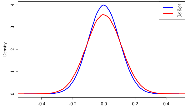
Kerndichteschaetzung des KQ und gewichteten Schaetzers
