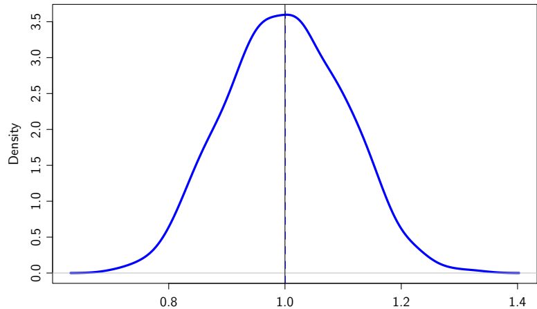
Kerndichteschaetzung des KQ Schaetzers gegeben X
