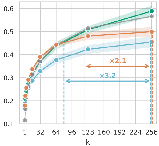
AIME 2024
