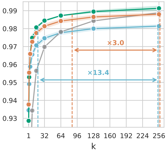
GSM8K
