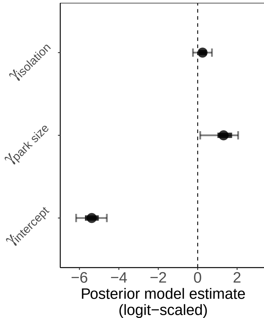
b) Colonization
