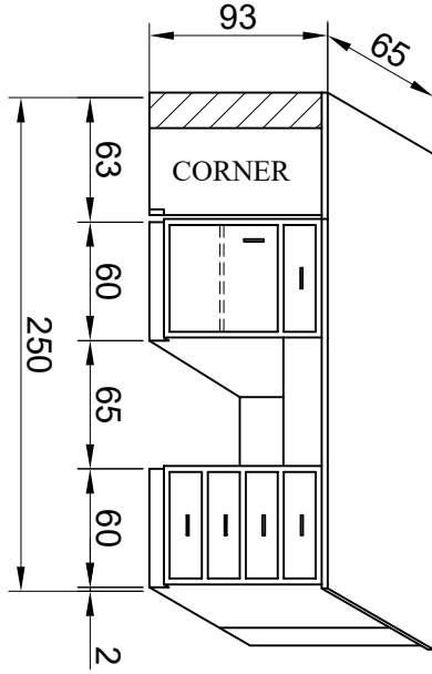
ELEVATION 'D'
