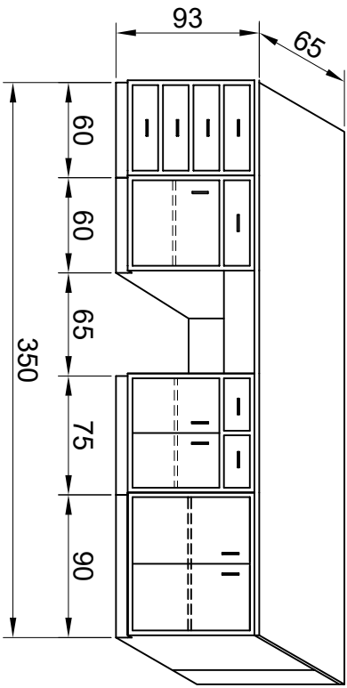
ELEVATION 'C'
