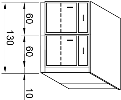
ELEVATION 'B'
