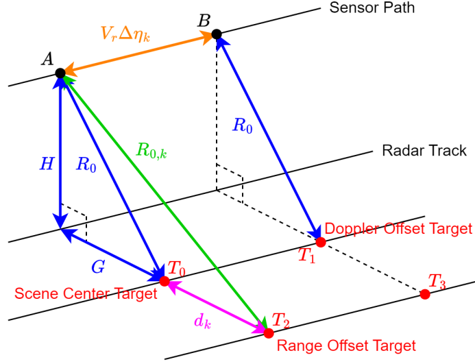
圖 7: 點散射體回波模型幾何關係示意圖。
