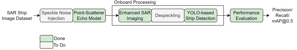
圖 2: 研究目標概念圖：由 SAR 船舶影像資料集出發，經 speckle noise 注入與點散射體回波模型模擬，送入星載（onboard）處理流程——強化 SAR 成像、去斑、YOLO 船舶偵測——最終產出 Precision/Recall/mAP@0.5 等效能指標（指標定義詳見 3.3 節）。圖中綠色標示已完成之工作項目，灰色標示尚未完成之項目。
