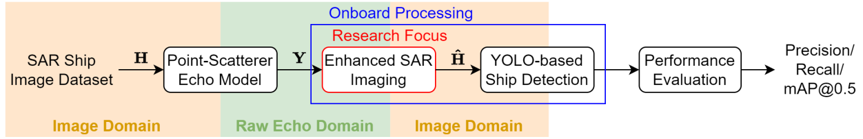
圖 2: 評估架構管線：點散射體回波模型 → 強化 SAR 成像（研究重點）→ YOLO 船舶偵測 → 效能評估。
