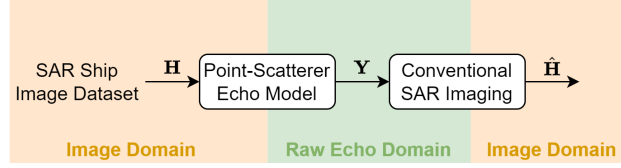
圖 6: 傳統 SAR 成像管線：點散射體回波模型 → 傳統 SAR 成像。
