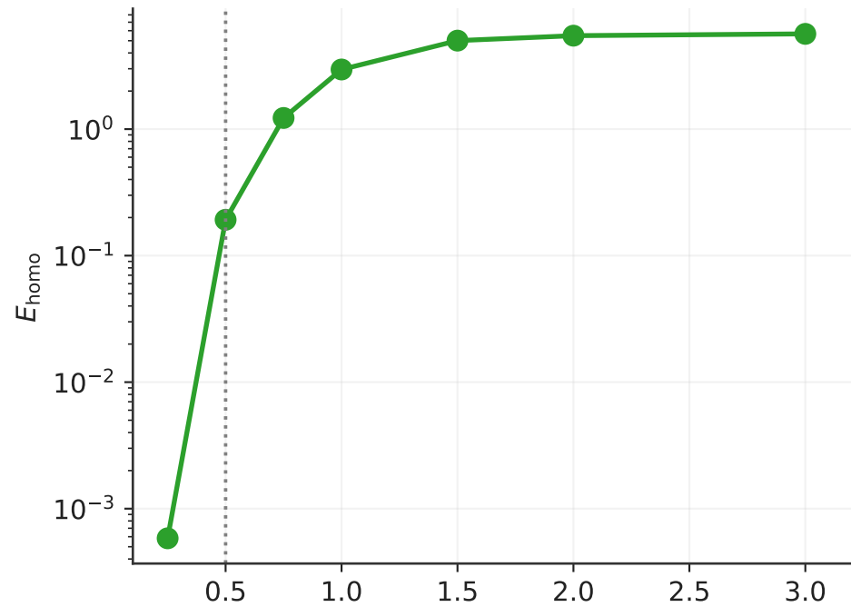
(d) Commutator gap (log)
