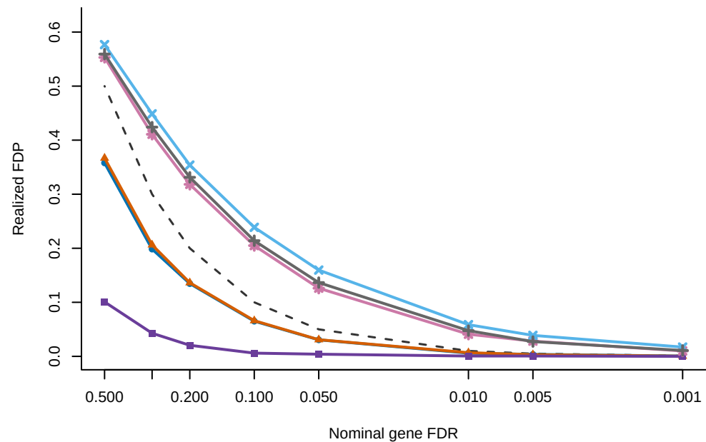
D Realized FDP: MOI 0.30
