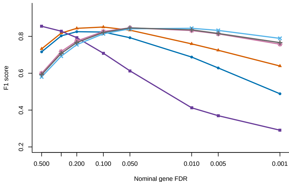
C F1: MOI 0.30
