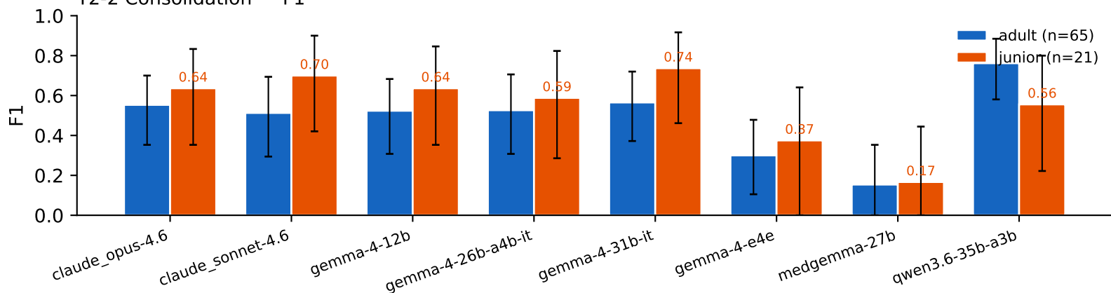
T2-2 Consolidation — F1
