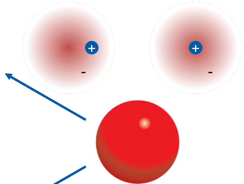
비극성 분자
