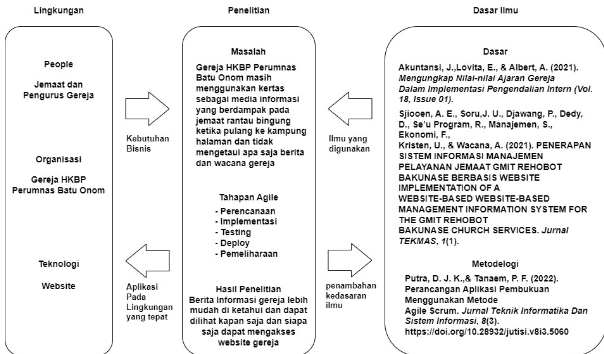
Gambar I.1 kerangka berfikir
