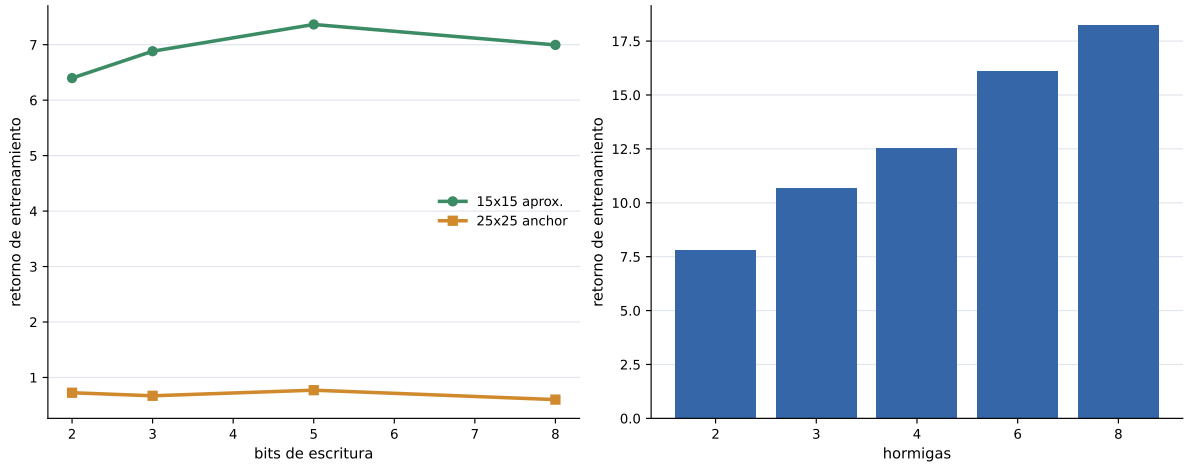
Figura 2: Comparación entre dos hipótesis tempranas. El panel izquierdo muestra retornos de entrenamiento al variar la cantidad de bits de escritura; el panel derecho muestra retornos al variar la cantidad de hormigas. La lectura favorece una explicación de cobertura multi-agente antes que una explicación basada solo en aumentar el alfabeto de escritura. Estas curvas no son evaluaciones held-out.
