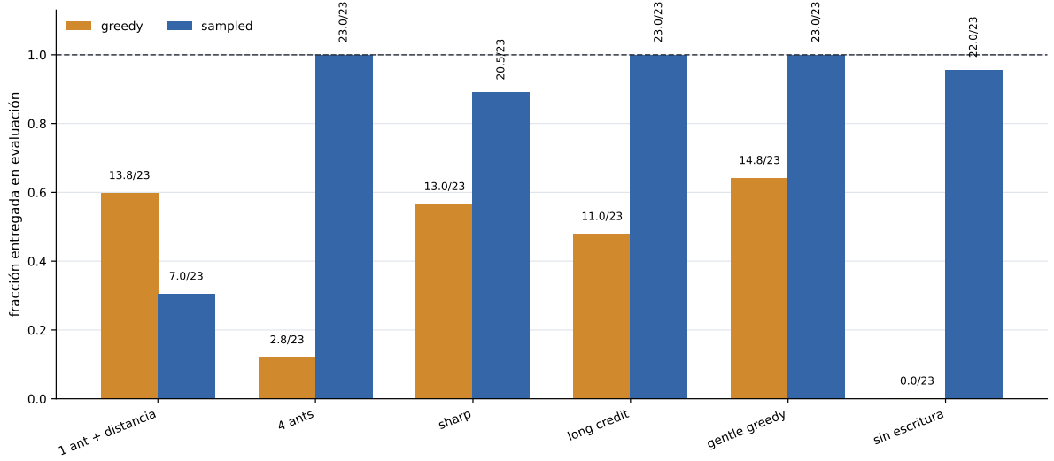
Figura 1: Evaluación 25x25 bajo dos protocolos de despliegue. Cada barra muestra la fracción de comida entregada y anota entregas sobre 23 unidades. La línea punteada marca la tarea completa: el resultado importante es la brecha entre movimiento greedy y movimiento muestreado, no solo el máximo alcanzado.
