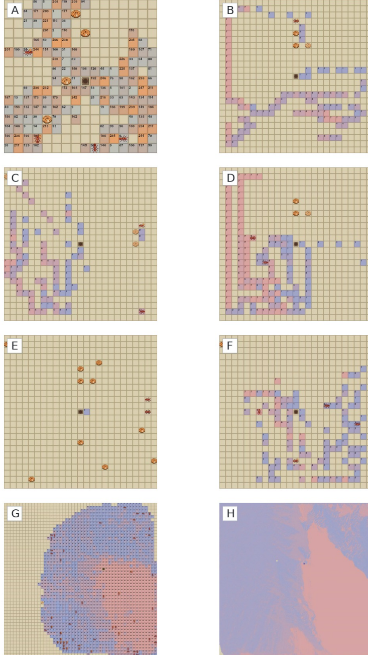
Figura 7: Fotogramas extraídos de videos locales. A: línea base aleatoria. B–F: progresión visual del currículo 25x25 con 2, 3, 4, 6 y 8 hormigas. G: frontera 50x50 con 60 hormigas. H: despliegue solo-actor 1000x1000 de la política 50x50. La figura no es evidencia cuantitativa; sirve para interpretar la semántica visual de las métricas.
