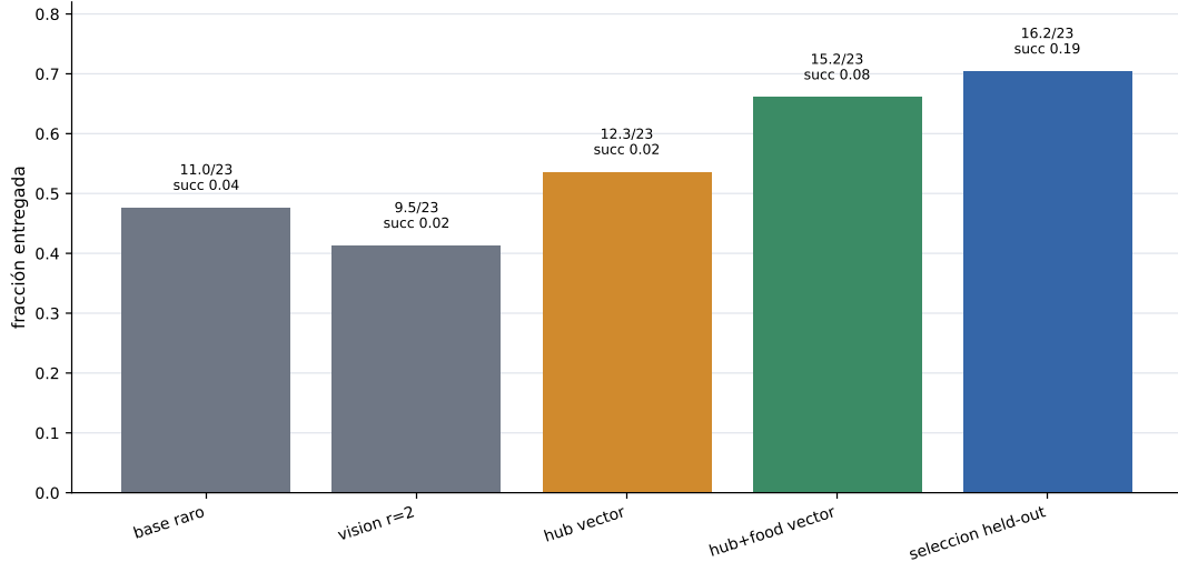
Figura 7: Evaluaciones seleccionadas en el escenario 50x50 con fuentes raras. Las barras reportan fracción entregada y anotan entregas sobre 23 junto con tasa de éxito. Las ayudas vectoriales parecen facilitar descubrimiento, pero la mejora no prueba comunicación emergente porque las corridas cambian más de una variable.
