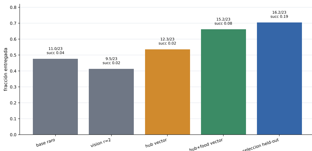
Figura 3: Evaluaciones seleccionadas en el escenario 50x50 con fuentes raras. Las barras reportan fracción entregada y anotan entregas sobre 23 junto con tasa de éxito. Las ayudas vectoriales parecen facilitar descubrimiento, pero la mejora no prueba comunicación emergente porque las corridas cambian más de una variable.
