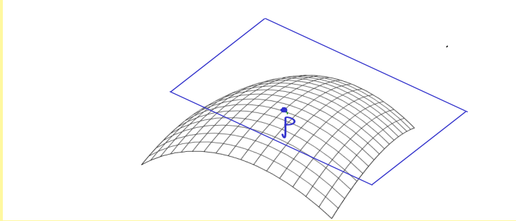
המישור הזה נקרא המישור המשיק למשטח בנקודה P .
