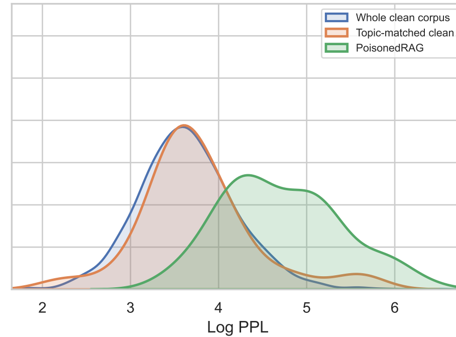
PoisonedRAG
