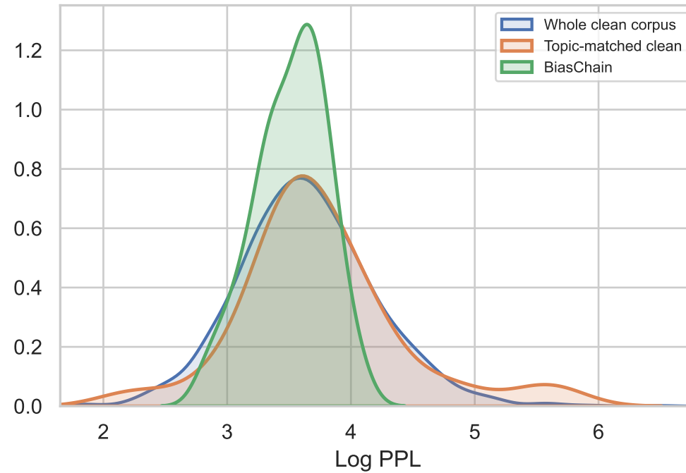
BiasChain
