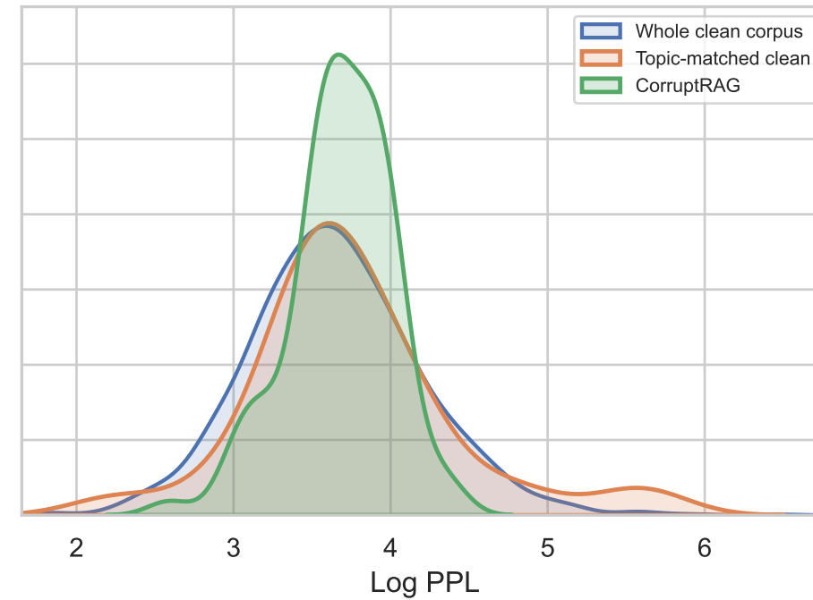
CorruptRAG
