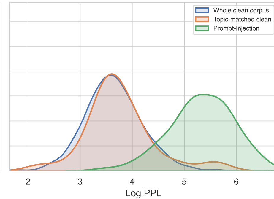
Prompt-Injection
