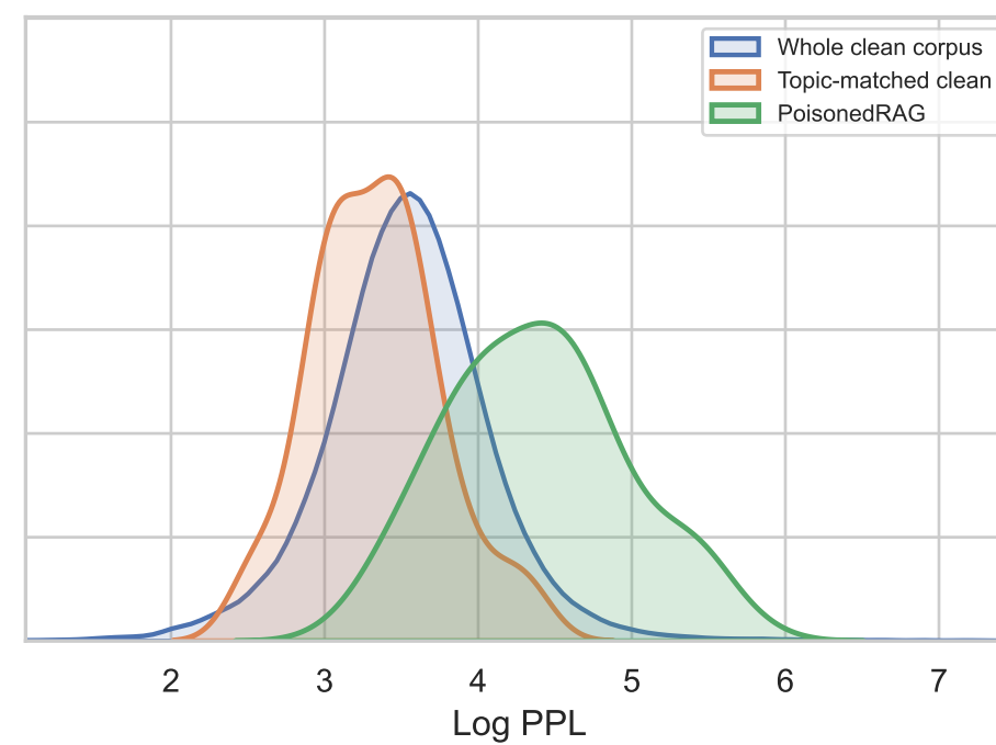
PoisonedRAG
