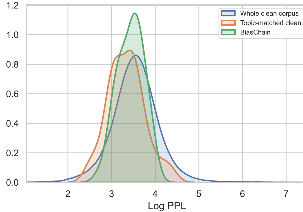
BiasChain
