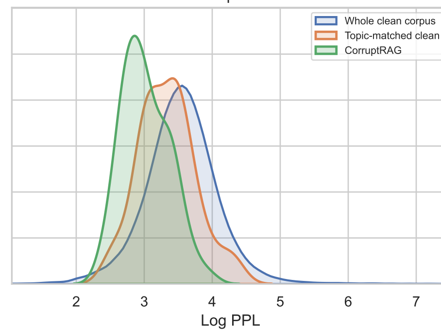
CorruptRAG
