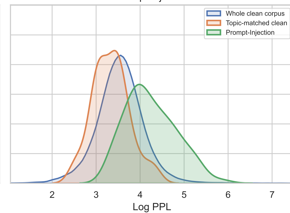
Prompt-Injection
