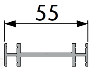
Montageprofiel
