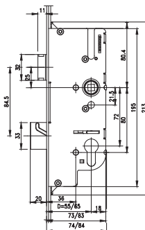
Maatvoering hoofdslootkast krukbediend
