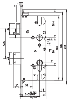
Maatvoering hoofdslootkast cilinderbediend
