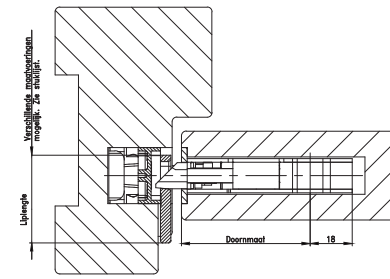
Doorsnede deur en kozijn
