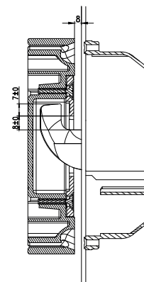
Detail sluithaak in sluitkom
