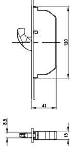
Haakschoot boven
