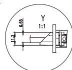
Haakschoot onder
