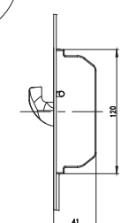
Haakschoot onder
