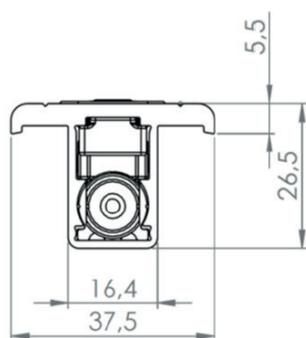
Dwarsdoorsnede NX-3809 DEUR
