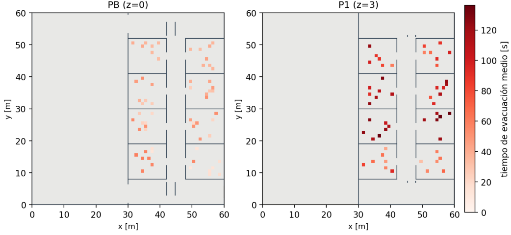
Figura 10: Tiempo de evacuación medio según la celda de origen ( N = 120 ). Las aulas de la planta alta (tonos oscuros) evacúan mucho más lento que las de la planta baja por tener que descender por las escaleras.
