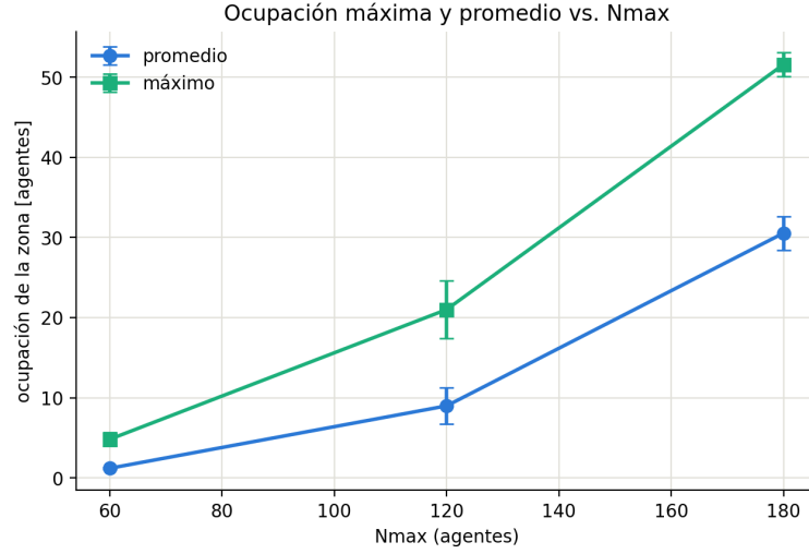
Figura 7: Ocupación máxima y promedio de la zona en función de N_{\text{máx}} .
