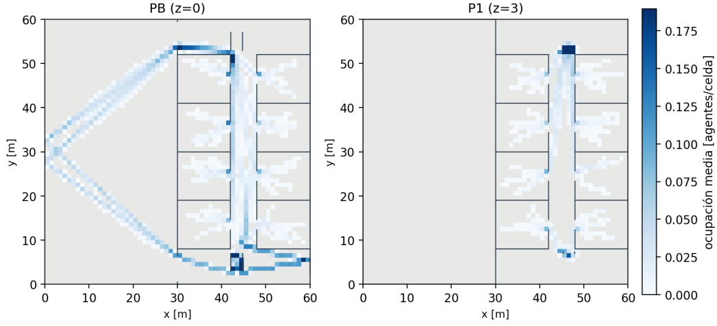
Figura 8: Densidad de ocupación durante la evacuación ( N = 120 ): el pasillo central y las escaleras concentran el flujo.
