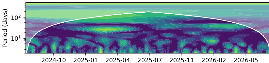
BUIDL vs. FANG: wavelet coherence
